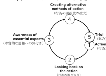
図1 ALACT モデル
